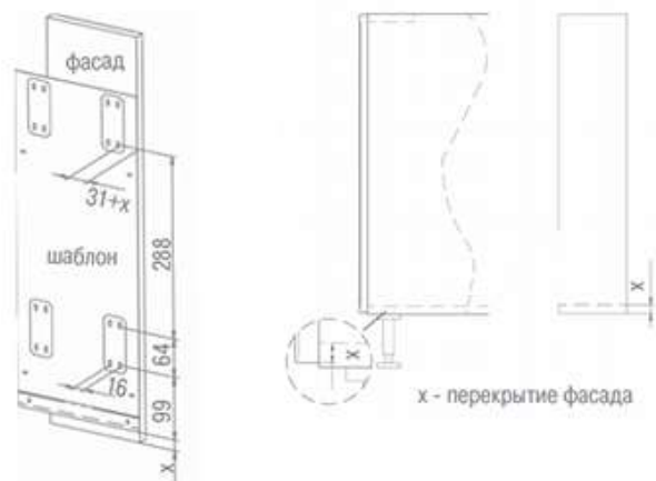
Присадочные размеры фасада
