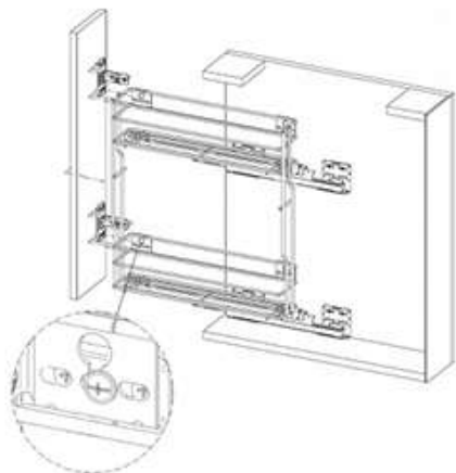
Установка фасада на корзину
